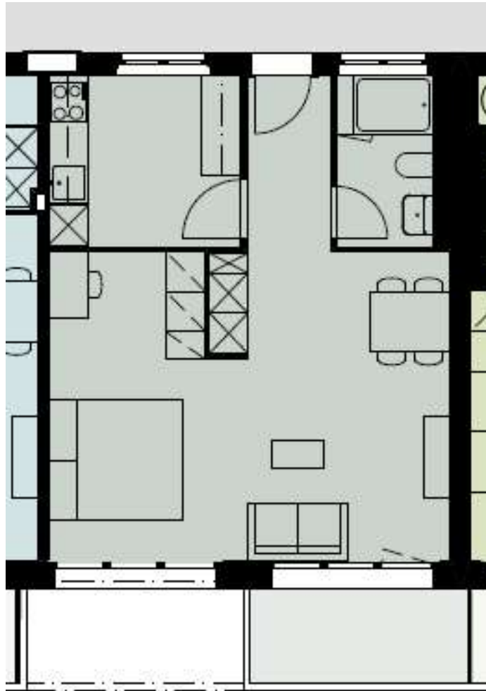
Whg. 4.3. 1.5-Zimmer-Wohnung NWF: 43.51 m 2
