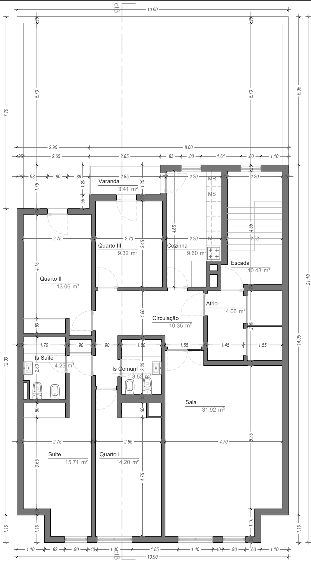
PLANTA DOS PISOS 2, 3, 4 E 5
